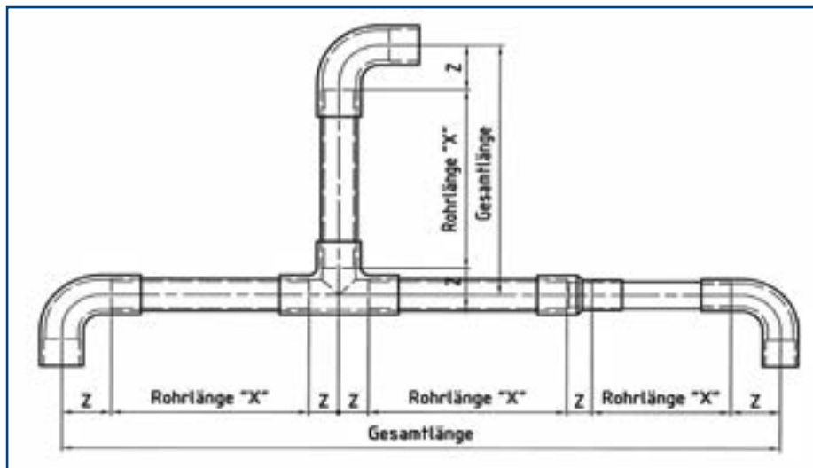
Ermittlung der Rohrlängen mittels Z-Maß-Methode
