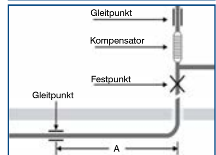
Dehnungsausgleich durch Rohrführung (Bilder: Deutsches Kupferinstitut e.V.)
