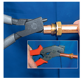
4. Hacer las muescas 4. Fazer as marcas no tubo
