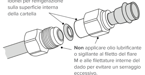
Raccordo cartellato in acciaio Inox e rondella cartellata in rame.
