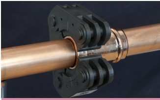
1. Inserire l'anello di pressatura
