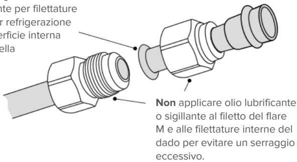
Raccordo cartellato in rame.
